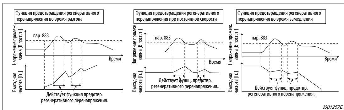
Рис. 6-262: Функция регенеративного перенапряжения.
