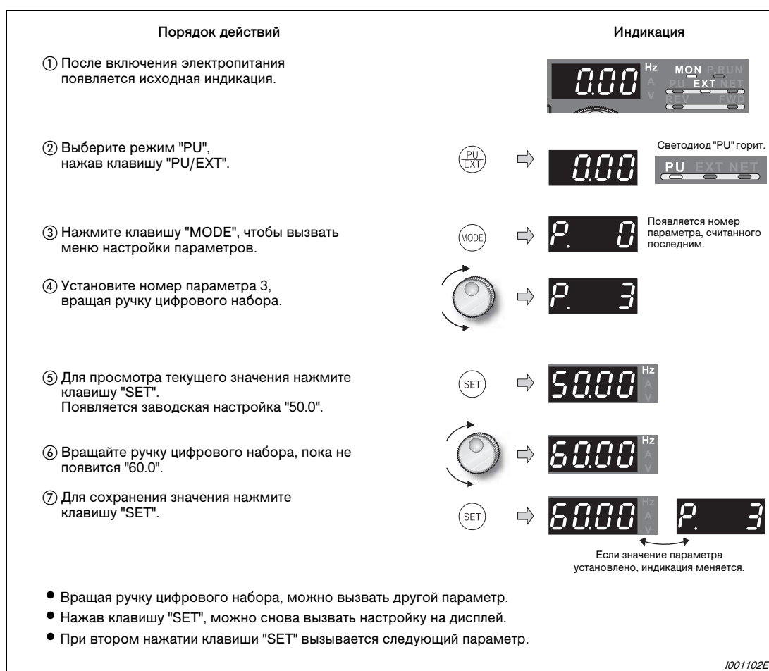
Рис. 5-2: Настройка базовой частоты
