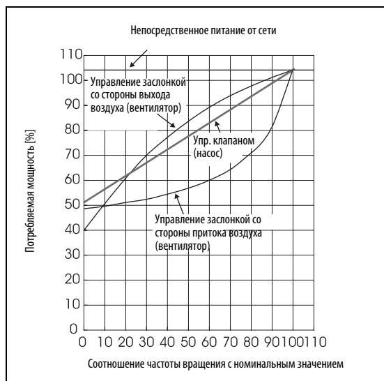
Рис. 6-174: Характеристики потребления мощности
