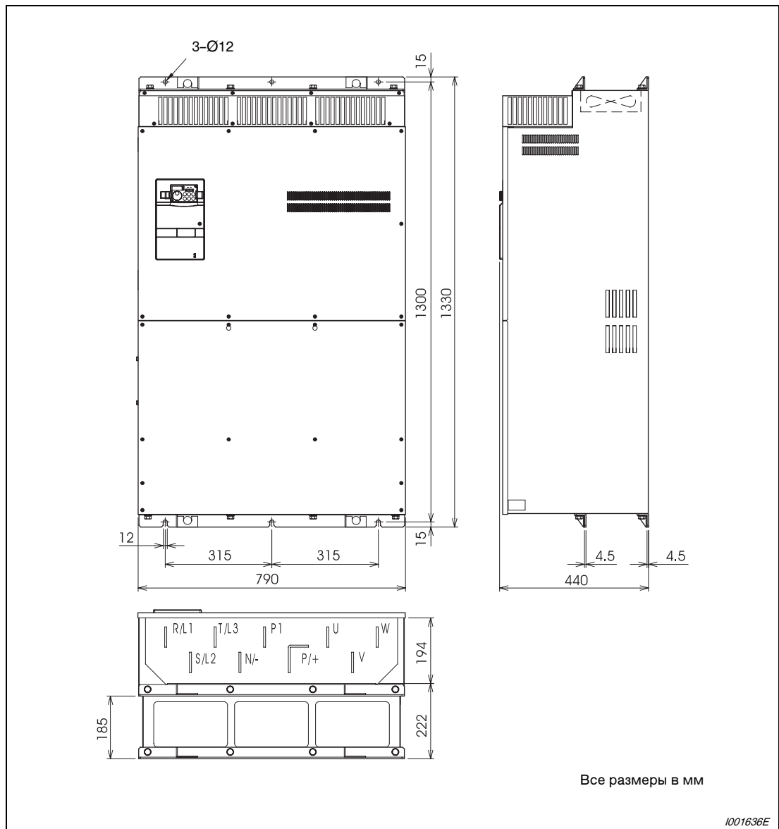
Рис. А-10: Размеры FR-A 740-07700 и FR-A 740-08660
