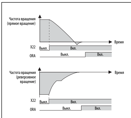
Рис. 6-121: Выполнение ориентации при левом вращении
