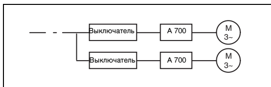
Рис. 3-2: Расположение силовых выключателей
