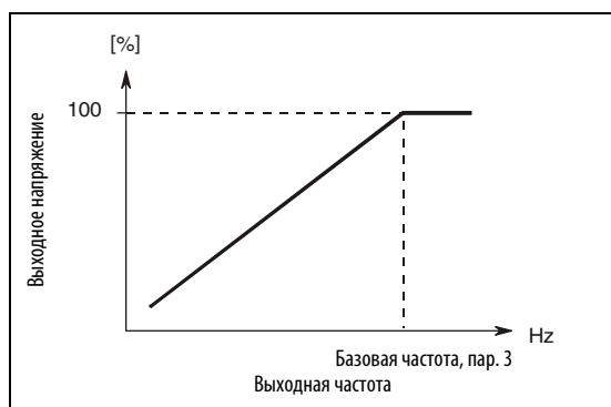
Рис. 6-60: Линейная характеристика
