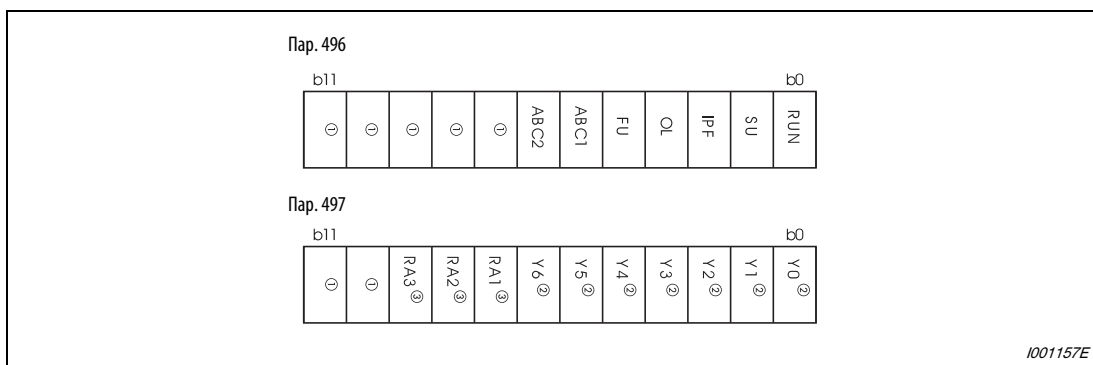
Рис. 6-141: Данные удаленного вывода
