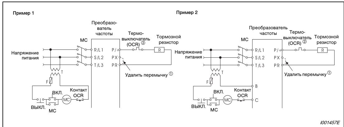
Рис. 3-33: Защитная схема
