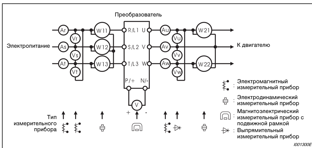
Рис. 7-7: Измерения на силовой части
