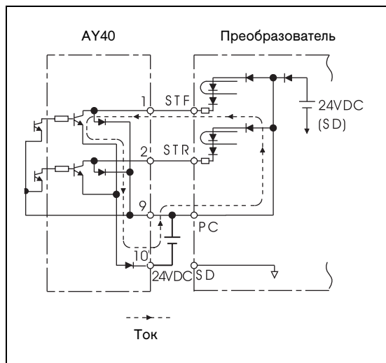
Рис. 3-15: Применение внешнего электропитания в сочетании с выходами программируемого контроллера
