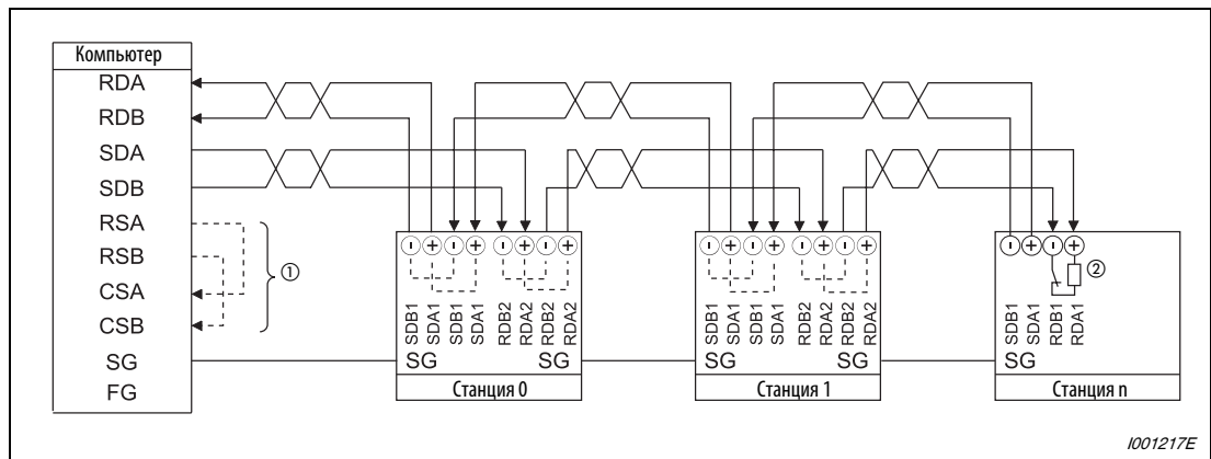
Рис. 6-219: Соединение с несколькими преобразователями частоты
