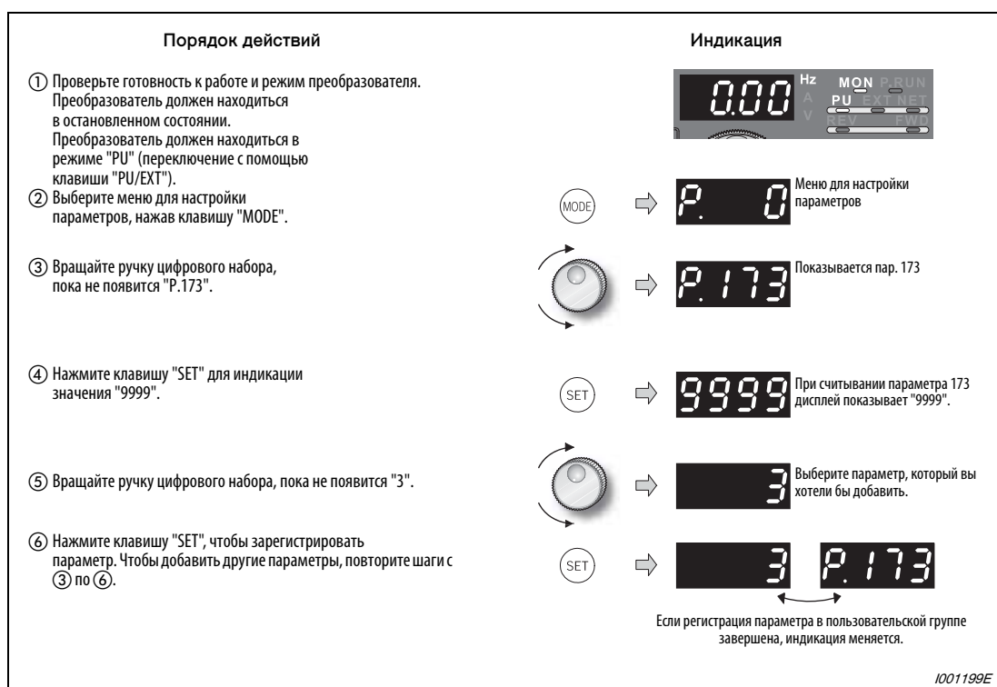
Рис. 6-200: Включение параметра 3 в пользовательскую группу
