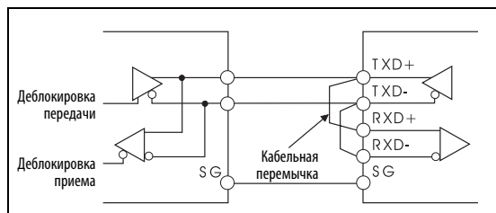
Рис. 6-220: Соединение по 2-проводной схеме
