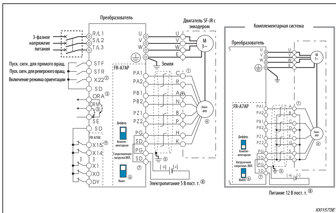
Рис. 6-113: Пример схемы
