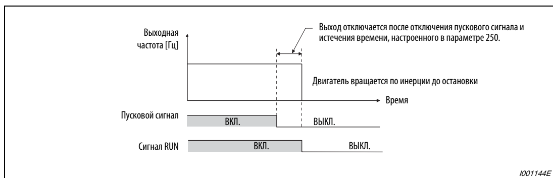
Рис. 6-106: Метод останова, если параметр 250 ≠ 8888 или 9999
