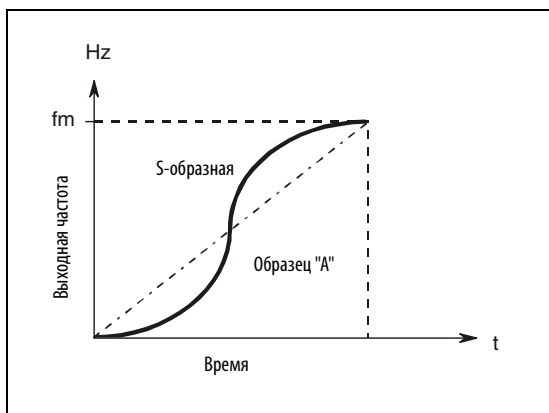
Рис. 6-81: Характеристика, если параметр 29 = "1"
