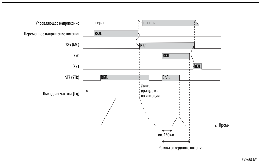
Рис. 6-101: Пример 1 работы при исчезновении сетевого напряжения
