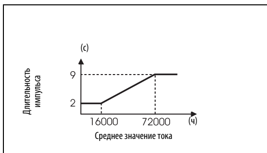
Рис. 6-270: Длительность импульса, отображающего значение счетчика интервала техобслуживания
