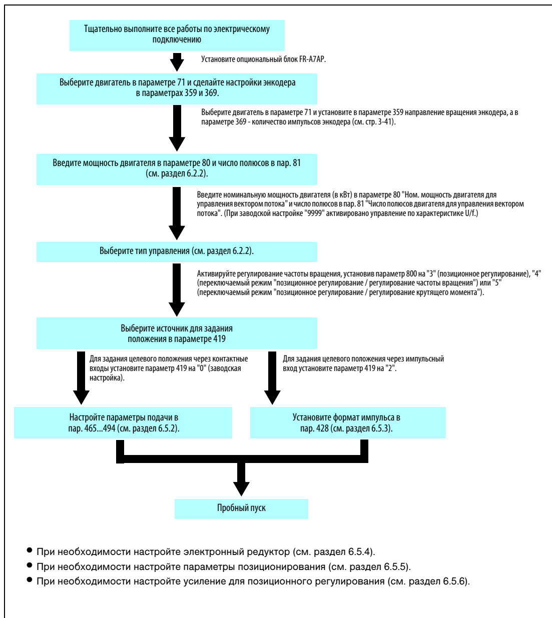
Рис. 6-37: Выбор позиционного регулирования
