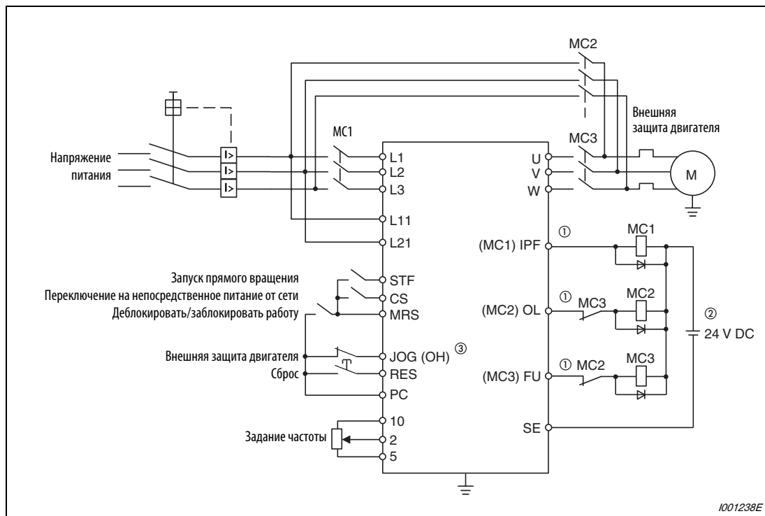
Рис. 6-248: Подключение силовых контакторов
