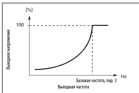
Рис. 6-61: Квадратическая характеристика
