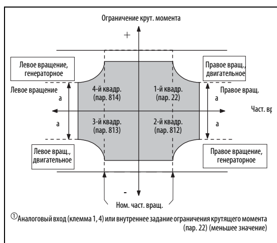
Рис. 6-9: Задание ограничения крутящего момента через аналоговый вход
