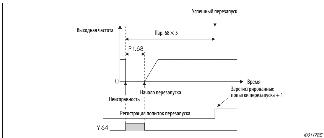
Рис. 6-169: Пример успешно выполненного перезапуска
