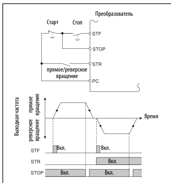
Рис. 6-130: Управление с помощью 3-проводной схемы (пар. 250 = 8888)
