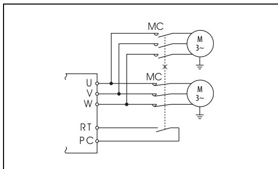
Рис. 6-89: Питание двух двигателей от одного преобразователя частоты
