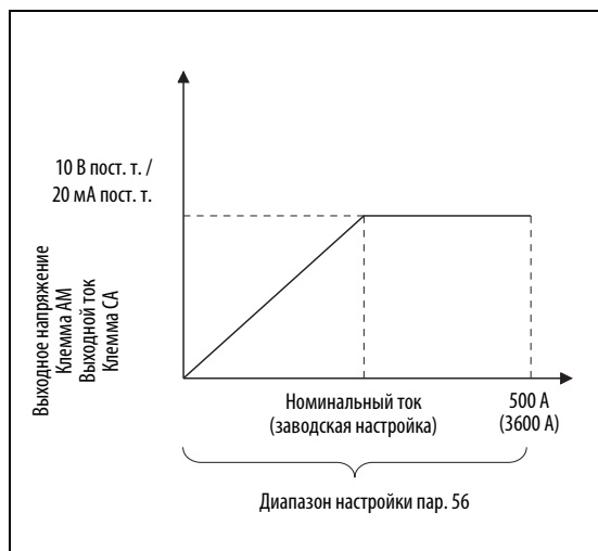
Рис. 6-149: Опорная величина для внешней индикации тока
