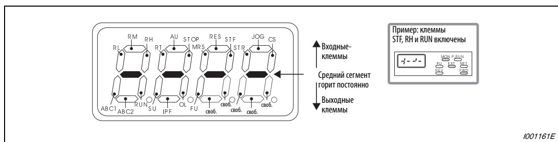
Рис. 6-145: Индикация состояний клемм ввода-вывода
