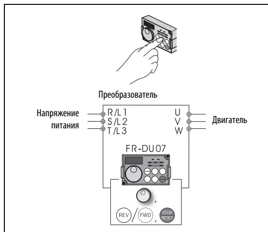
Рис. 6-206: Пулты управления
