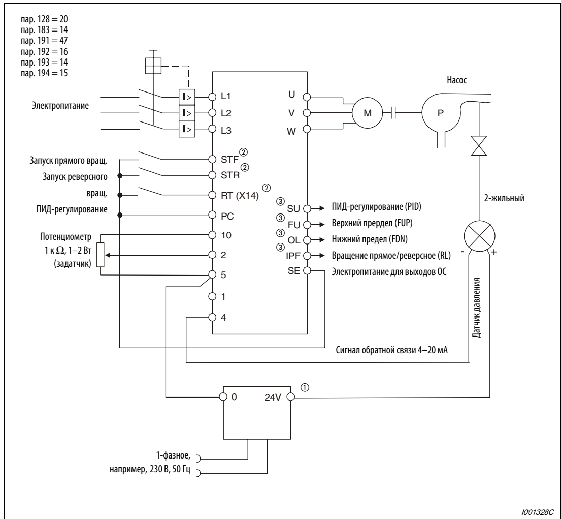
Рис. 6-242: Пример подключения при положительной логике
