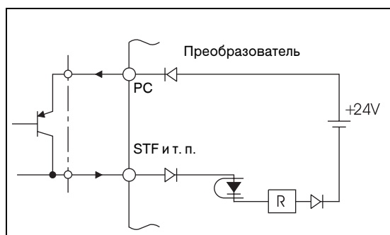
Рис. 3-19: Управление с помощью транзистора при положительной логике
