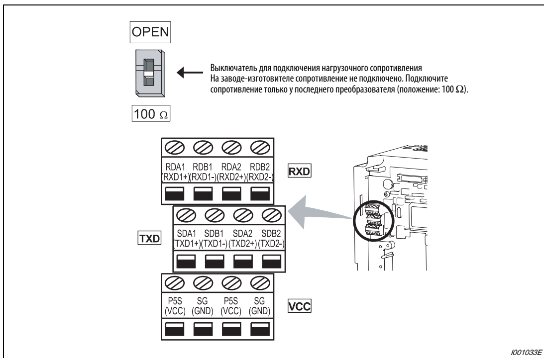
Рис. 6-214: 2-й последовательный интерфейс преобразователя
