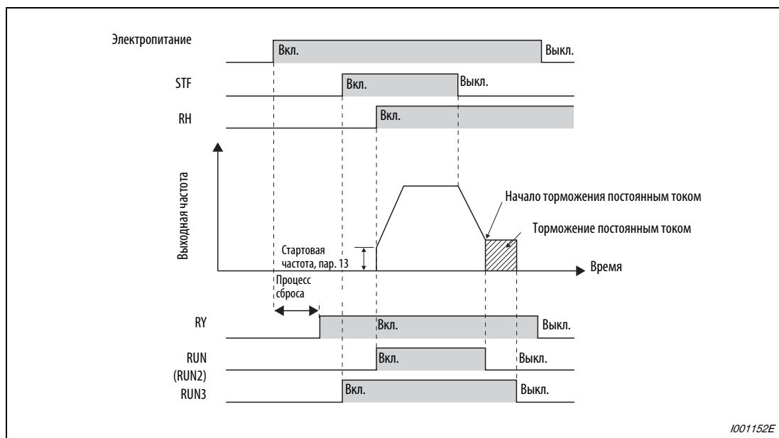
Рис. 6-131: Готовность к работе и вращение двигателя
