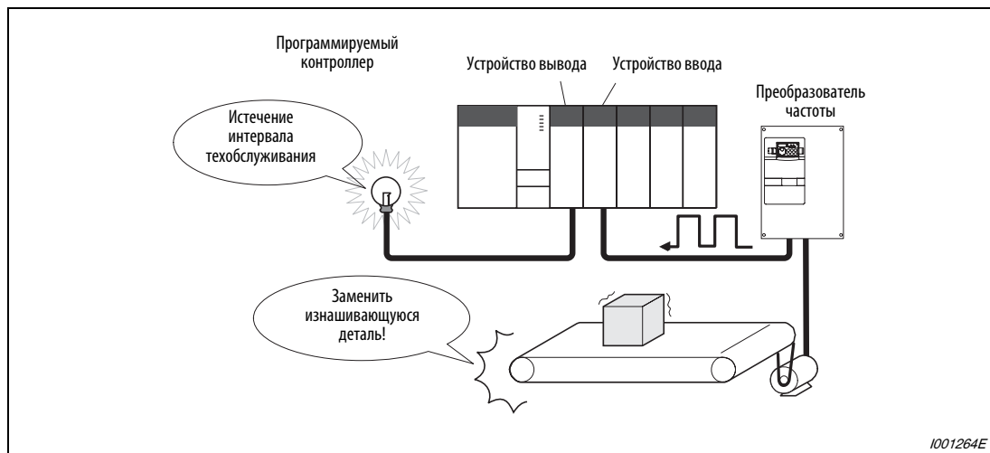
Рис. 6-267: Контроль интервала техобслуживания и среднего значения тока
