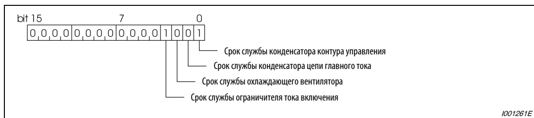
Рис. 6-265: Значение битов параметра 255
