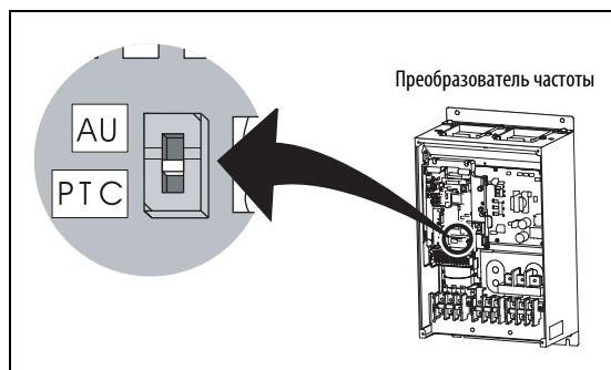
Рис. 6-93: Переключатель AU/PTC
