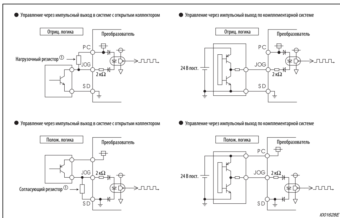
Рис. 6-258: Импульсный вход
