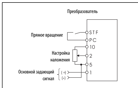
Рис. 6-182: Пример схемы для процентного наложения
