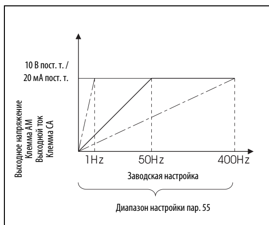
Рис. 6-148: Опорная величина для внешней индикации частоты
