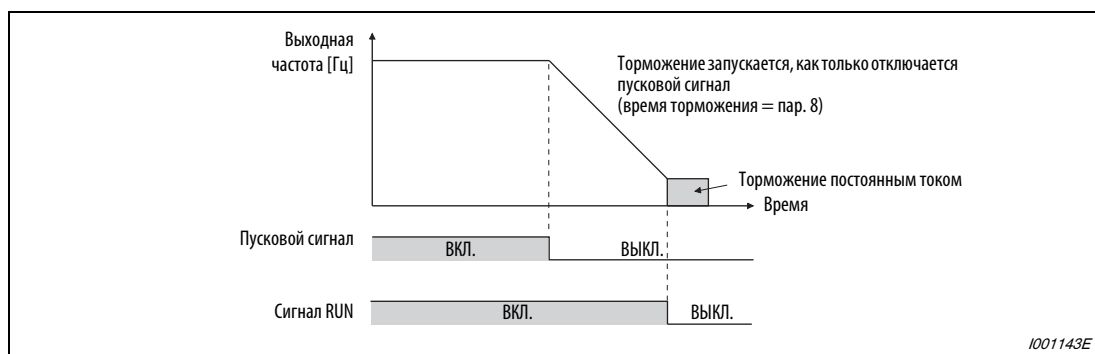
Рис. 6-105: Метод останова, если параметр 250 = 8888 или 9999
