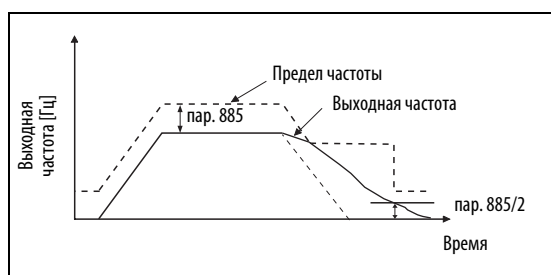
Рис. 6-263: Ограничение выходной частоты
