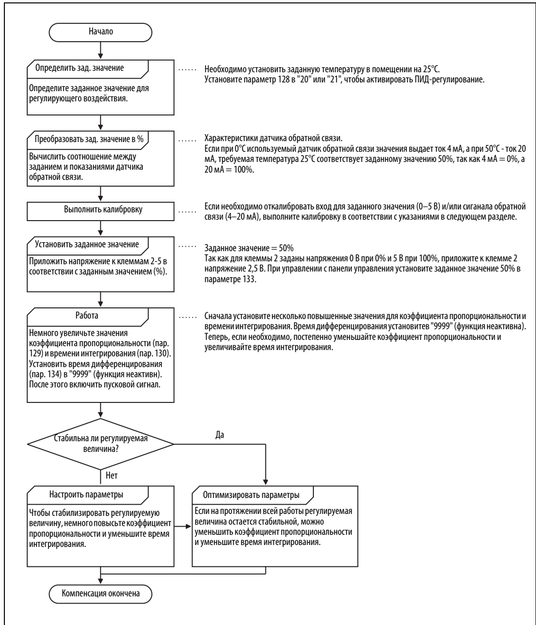
Рис. 6-246: Пример калибровки
