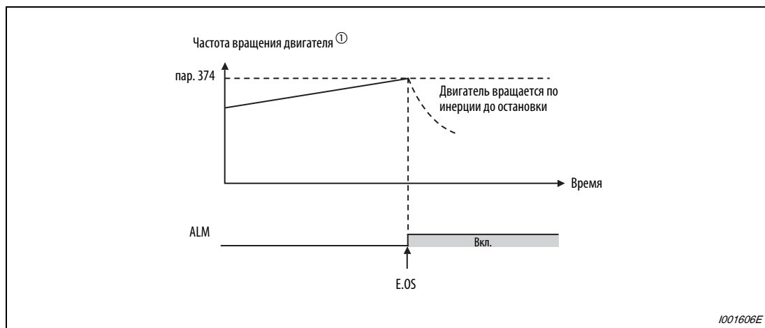
Рис. 6-171: Предел частоты вращения и вывод тревожной сигнализации
