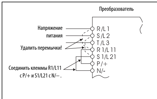
Рис. 6-163: Подключение
