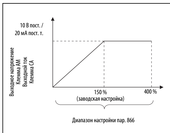
Рис. 6-150: Опорная величина для внешней индикации крутящего момента
