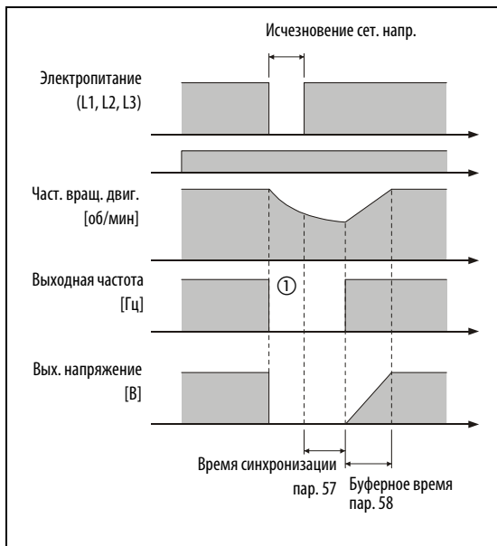
Рис. 6-159: Управление по характеристике U/f и расширенное управление вектором потока
