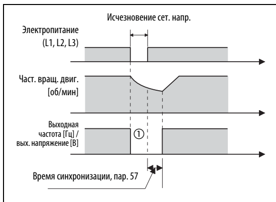
Рис. 6-160: Бессенсорное векторное управление
