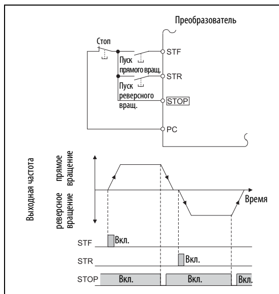
Рис. 6-129: Управление с помощью 3-проводной схемы (пар. 250 = 9999)
