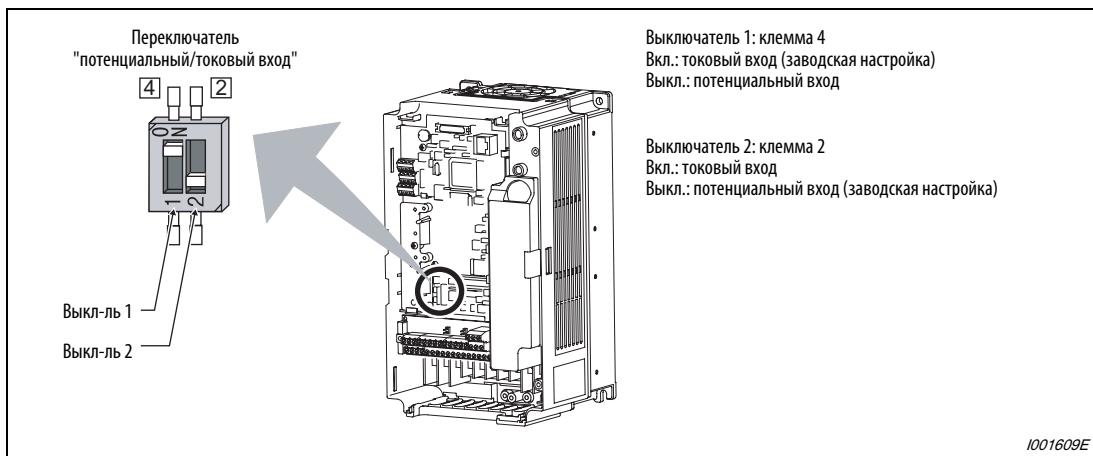
Рис. 6-175: Переключатель "потенциальный/токовый вход"
