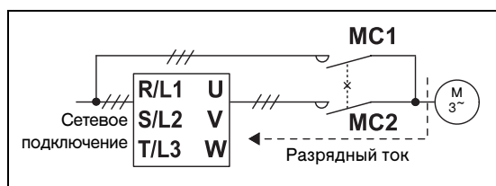
Рис. 4-1: Механическая блокировка силовых контакторов
