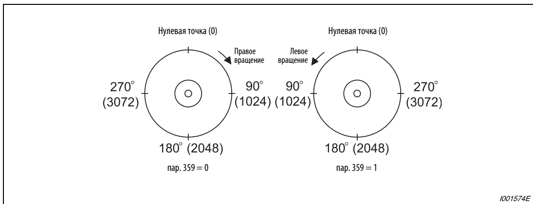
Рис. 6-114: Распределение адресов энкодера
