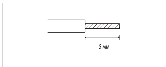
Рис. 6-215: Подготовка кабеля
