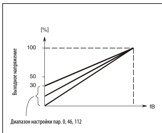
Рис. 6-45: Выходная частота относительно выходного напряжения
