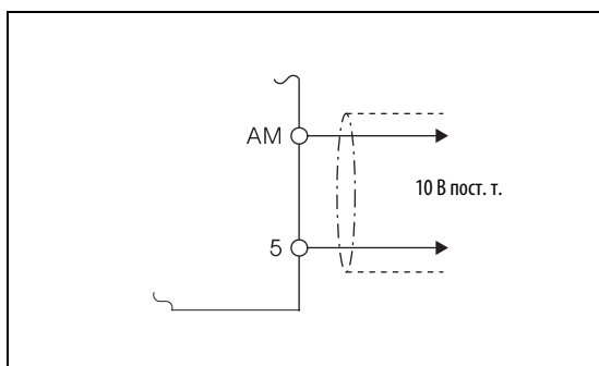
Рис. 6-153: Подключение аналогового прибора индикации к выходу АМ
