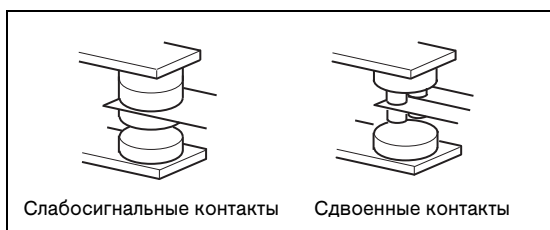
Рис. 3-20: Виды контактов
