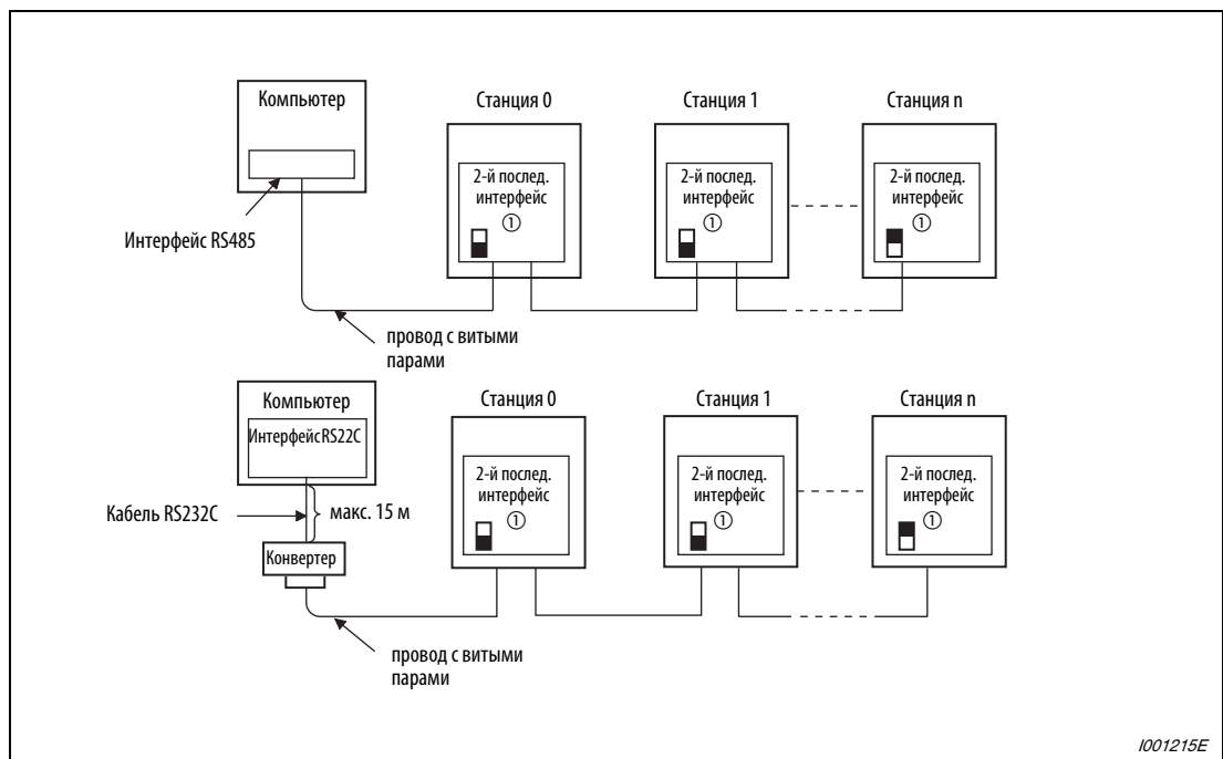
Рис. 6-217: Соединение с несколькими преобразователями частоты
