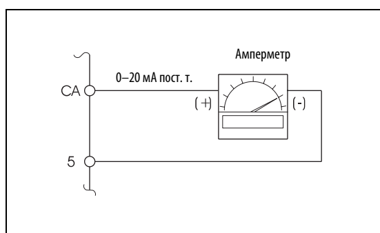
Рис. 6-151: Подключение аналогового измерительного прибора к выходу СА
