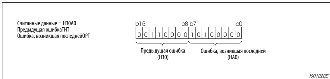
Рис. 6-229: Пример считывания данных аварийного сообщения
