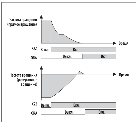
Рис. 6-120: Выполнение позиционного регулирования при прямом вращении
