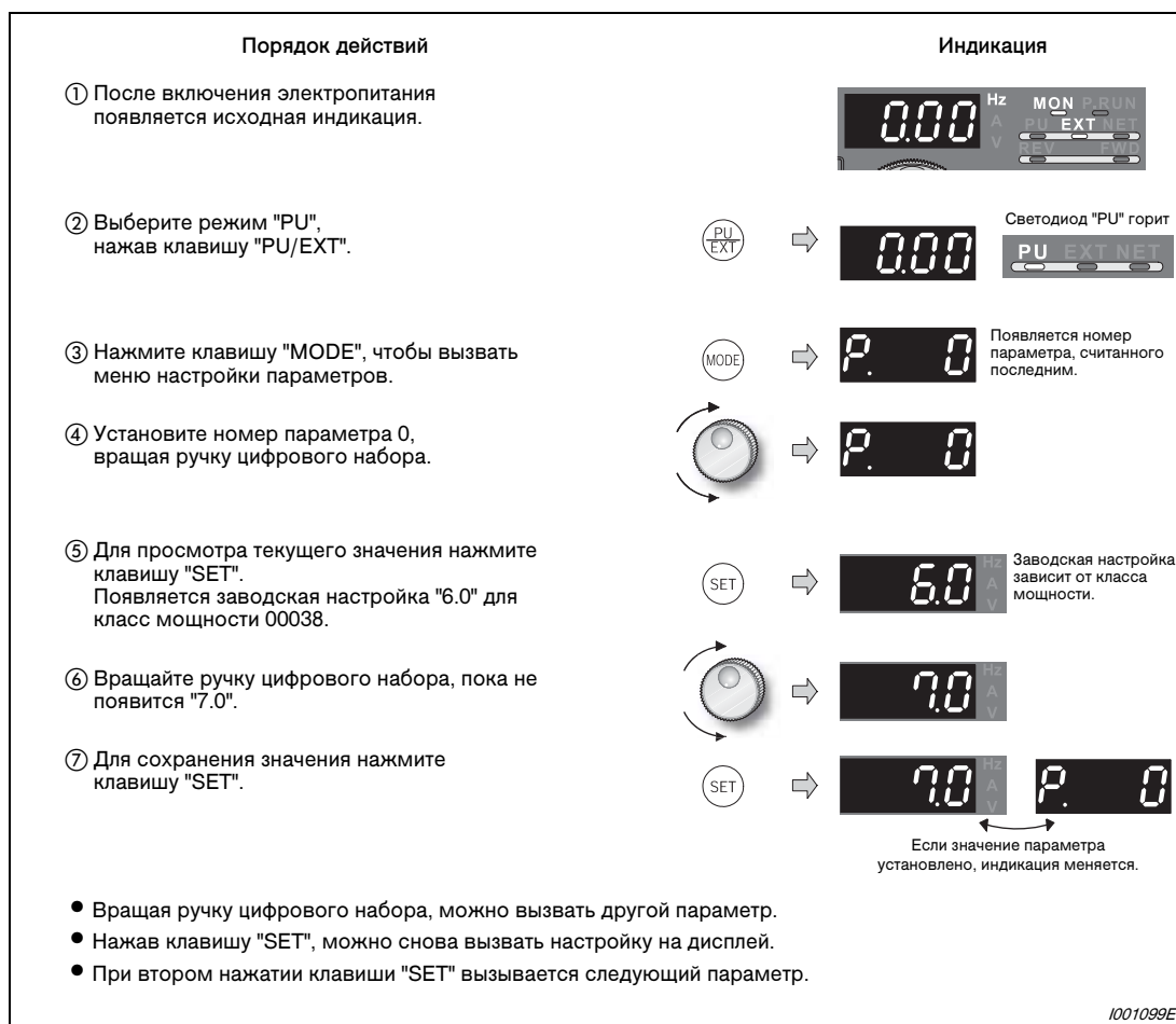
Рис. 5-4: Настройка пускового крутящего момента
