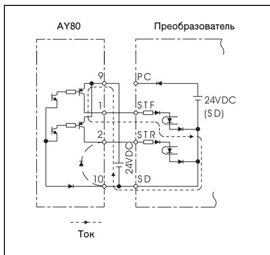
Рис. 3-16: Применение внешнего электропитания в сочетании с выходами программируемого контроллера
