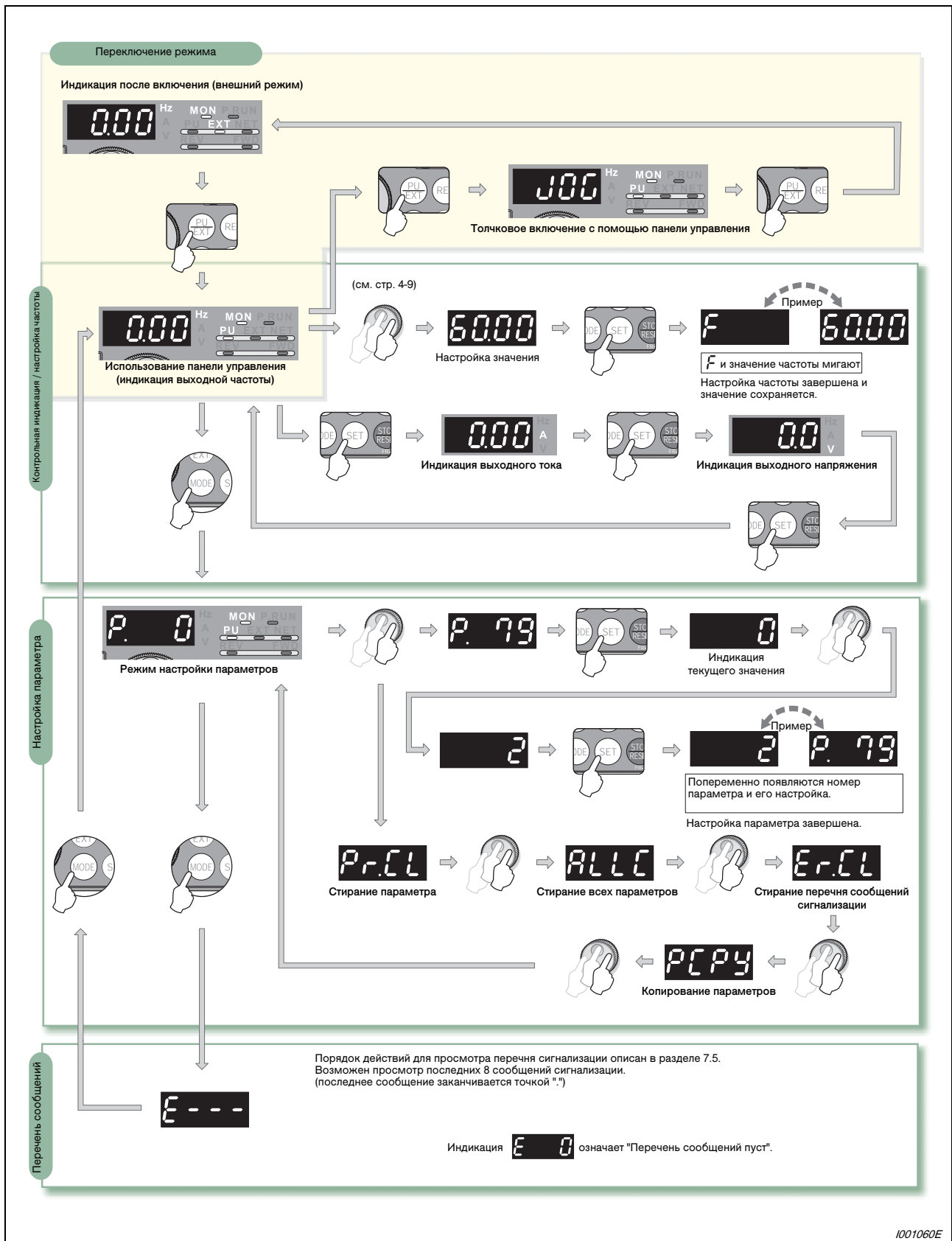
Рис. 4-4: Обзор основных функций панели управления FR-DU07
