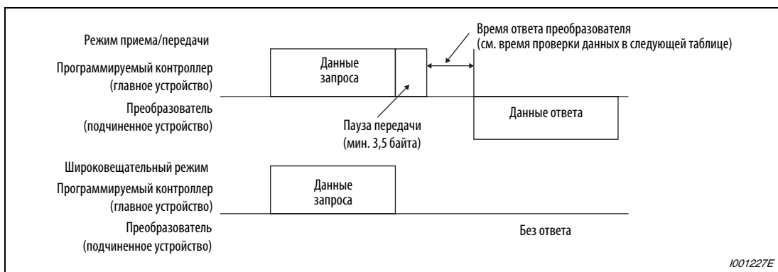
Рис. 6-230: Формат сообщений
