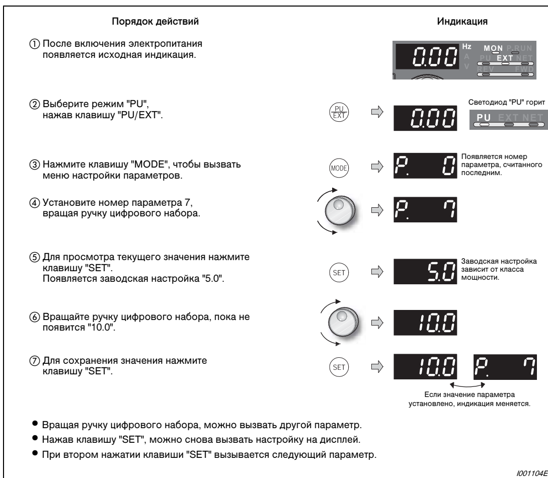
Рис. 5-8: Настройка времени разгона
