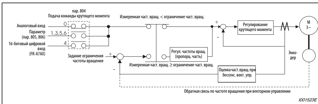
Рис. 6-26: Блок-схема
