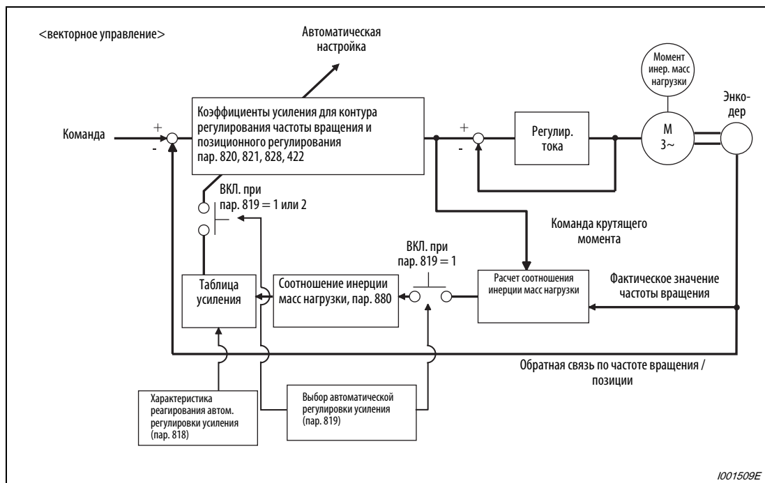
Рис. 6-15: Блок-схема автоматической настройки усиления
