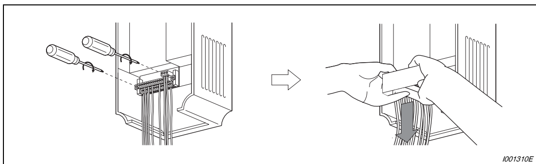
Рис. 8-12: Демонтаж клеммной колодки
