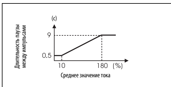
Рис. 6-269: Длительность паузы между импульсами, отображающей среднее значение тока
