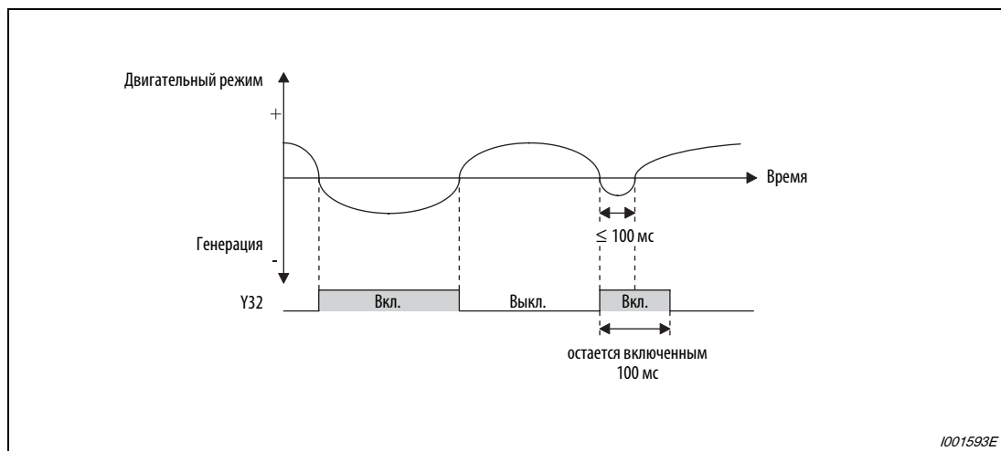
Рис. 6-134: Генераторный режим
