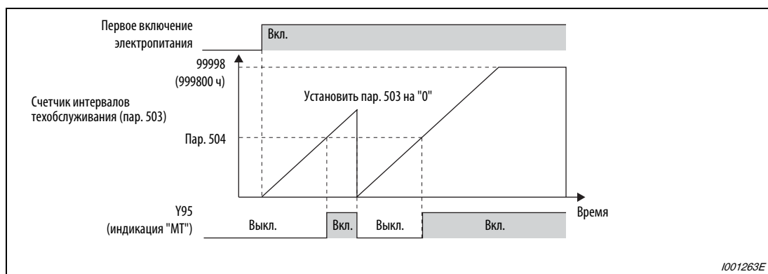
Рис. 6-266: Счетчик интервалов техобслуживания
