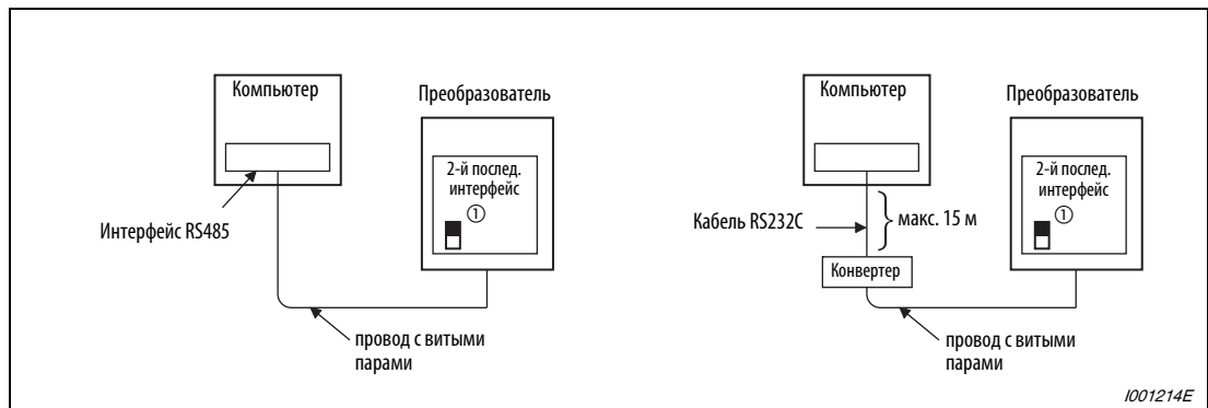
Рис. 6-216: Соединение с одним преобразователем частоты
