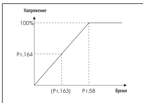
Рис. 6-162: Подъем напряжения при автоматическом перезапуске
