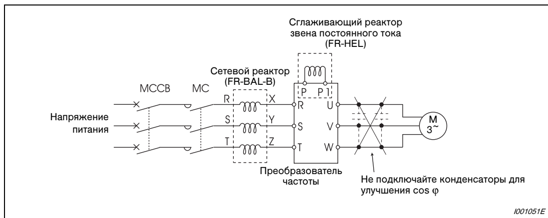
Рис. 3-52: Подавление высших гармоник в сетевых проводах
