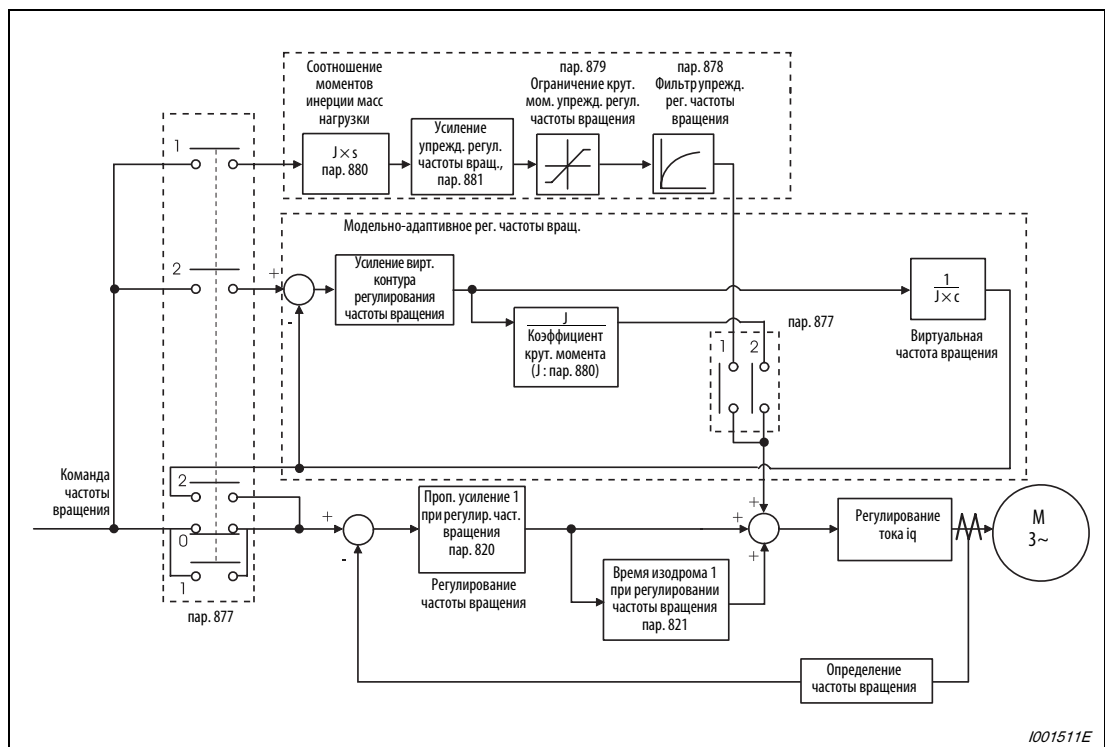
Рис. 6-19: Блок-схема
