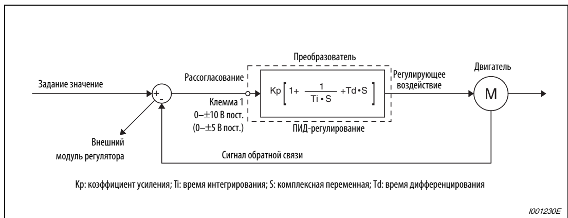
Рис. 6-235: Конфигурация системы для пар. 128 = 10, 11 (использование задания в виде рассогласования)
