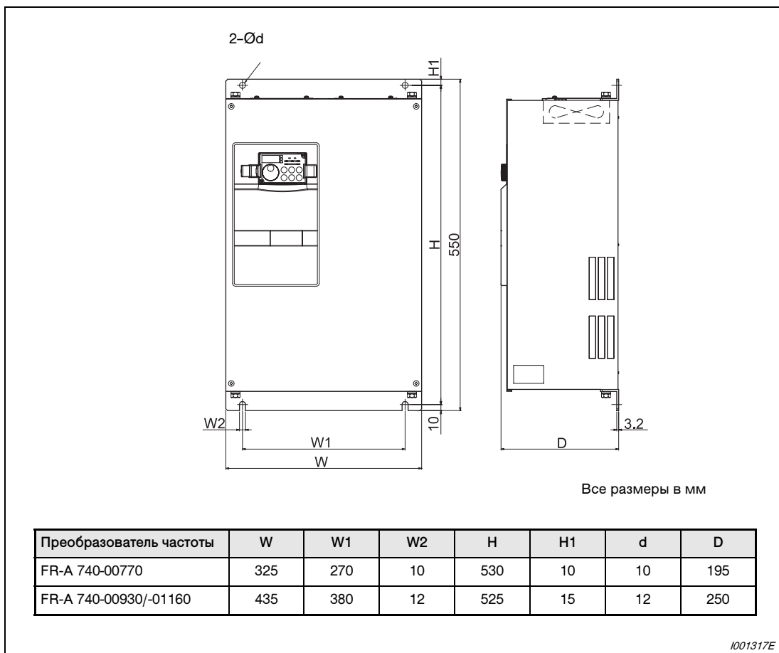
Рис. А-4: Размеры FR-A 740-00770 ... -01160
