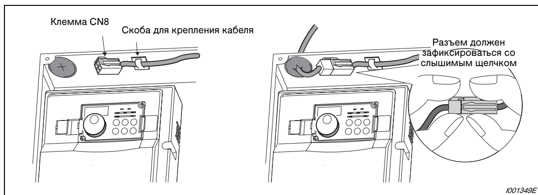
Рис. 3-38: Подключение клеммы CN8
