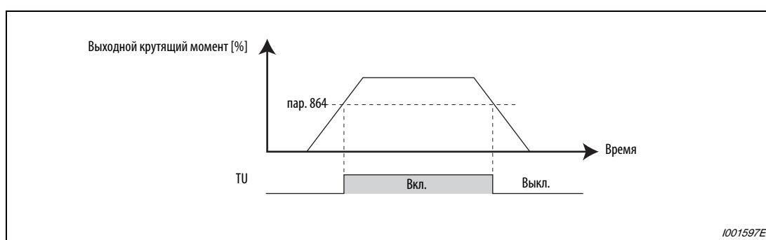
Рис. 6-140: Контроль крутящего момента
